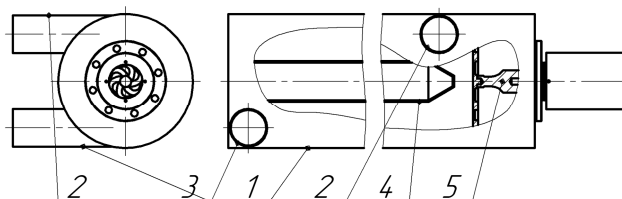
1 – коагуляционно-сепарационная камера; 2 – входной патрубок (закручиватель); 3 – выходной патрубок (раскручиватель); 4 – обтекатель (вытеснитель); 5 – дисковый излучатель;
