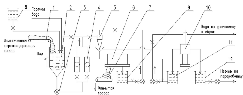
Рис. 5. АТС переработки нефтесодержащих грунтов с использованием УЗ техники: 1 – транспортёр нефтесодержащей породы, 2 – смеситель, 3 – насосный блок, 4 – УЗ реактор, 5 – гидроциклон, 6 – центрифуга, 7 – транспортёр отмытой породы, 8 – ёмкость химического реагента, 9 – сборник промывного фугата, 10 – сепаратор, 11 – сборник очищенной воды, 12 – сборник нефтепродуктов
