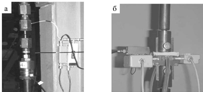
Рис. 1. Вертикальное (а) и горизонтальное (б) крепления датчиков АЭ на узлах деформационной машины 2167P – 50
