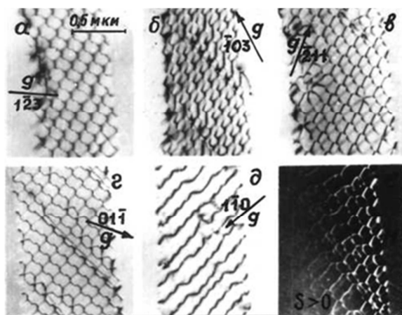
Рис. 1. Электронная микроскопия сетки из дислокаций пяти типов с разными векторами Бюргерса в молибдене [1].
