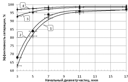
1 – ВЗП; 2 – агломератор (без УЗ) и ВЗП (без УЗ); 3 – агломератор (+УЗ) и ВЗП (без УЗ); 4 – агломератор (+УЗ) и ВЗП (+УЗ)
