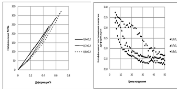
Рис. 2. Зависимость напряжения от деформации и для пятидесятих циклов нагружения и зависимость коэффициента поглощения упругой энергии от числа циклов нагружения для напряжений 0,6 \cdot \sigma_{0,2} ; 0,7 \cdot \sigma_{0,2} и 0,8 \cdot \sigma_{0,2} .
