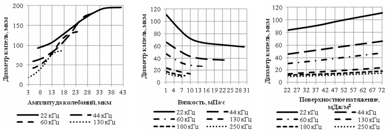
Рис. 2. Зависимости диаметра формируемых капель (мкм) жидкости от амплитуды колебаний (мкм) (а), поверхностного натяжения (мН/м) (б) и амплитуды колебаний (мкм) (в) при различных частотах (кГц)
