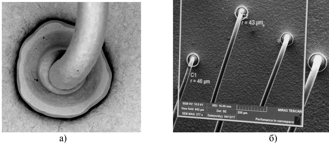
Рис. 3. Вид соединений шариком встык при использовании ультразвуковой частоты 64 кГц а) и ультразвуковой частоты 110 кГц б).
