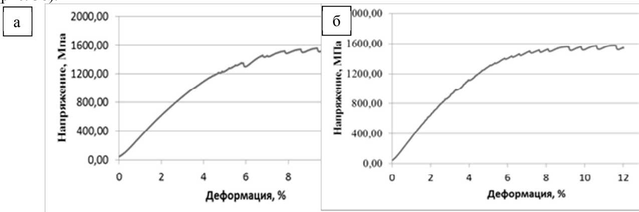
Рис. 3. Зависимости «напряжение-деформация» при растяжении с одиночным импульсным током сплава Ti-50,4at.%Ni после волочения: а) после предварительного волочения без УЗО; б) подвергнутого предварительному волочению с УЗО.
