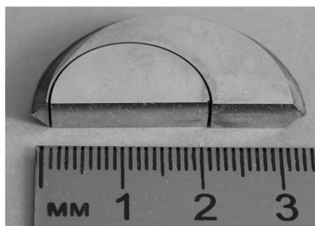
Рис. 2. Никелевый образец в форме полудиска с радиусом 10 мм, вырезанный из половины образца, деформированного кручением под давлением.
