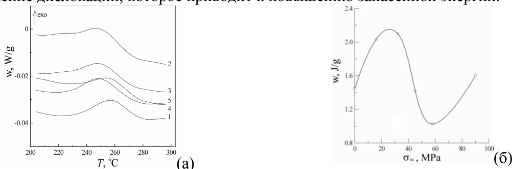
Рис. 1. (а) - Результаты ДСК: пики, связанные с процессами возврата в образцах никеля, подвергнутых КГД (1) и УЗО с амплитудами 15 (2), 30 (3), 45 (4), 60 (5) и 90 МПа (6); (б) - Зависимость значений запасенной энергии, выделившейся при проведении ДСК, от амплитуды УЗО
