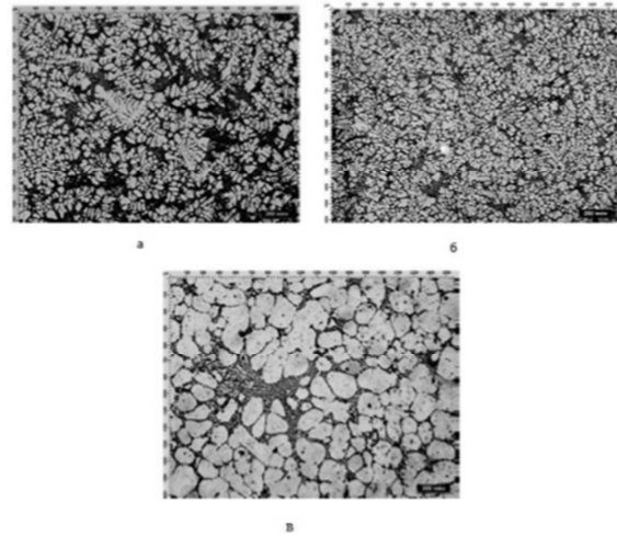
Рис. 2. Влияние УЗО на дендритную структуру сплава АК7 в эксперименте №1: а – исходное состояние; б - УЗО в течение 6 мин в интервале 607 – 600°C; в – УЗО в течение 6 мин при 600°C (x20), травлено
