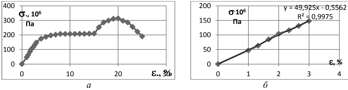
Рис. 2. Экспериментальная кривая, полученная с использованием разрывной машины (а-общая кривая, б-область чисто упругих деформаций)
