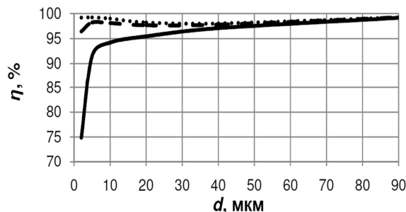
— Без УЗ ..... С УЗ 150 дБ — С УЗ 145 дБ Рис. 7. – Фракционная эффективность скруббера Вентури при различных уровнях звукового давления
