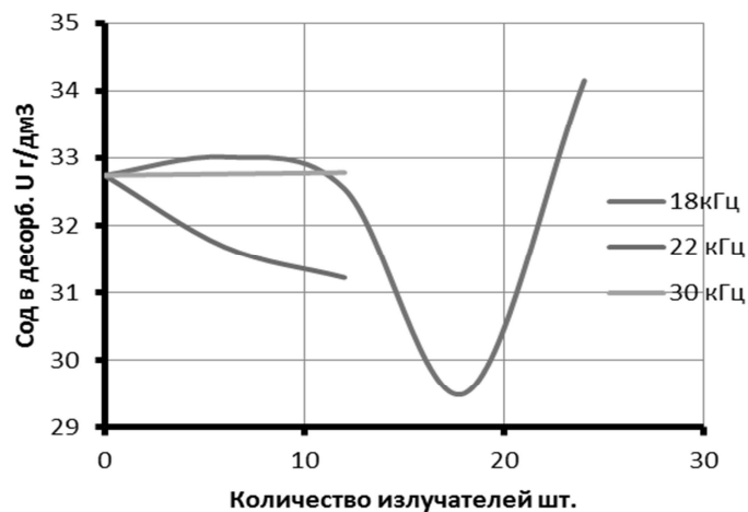
Рис. 2 - Изменение содержания урана в десорбате в зависимости от количества работающих излучателей
