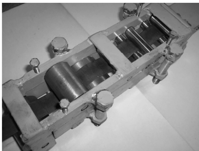
Рис. 1. Фото модели установки с заправленной полосой
