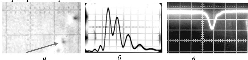
Рис. 2. Выявление и характеристика дефектов в стеклах АМД-методами (а - акустическое изображение трещины субмикронного размера в К-108; масштаб 11 мкм/дел.; б - изменение формы V(Z)-кривых в стекле в районе микротрещины; в – выявление микротрещины в режиме строки (по вертикали 1 дел. = 0,25 В, по горизонтали 1 дел. = 8 мкм)
