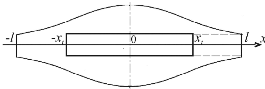
Рис.1. Принципиальная схема двухампульного волновода
