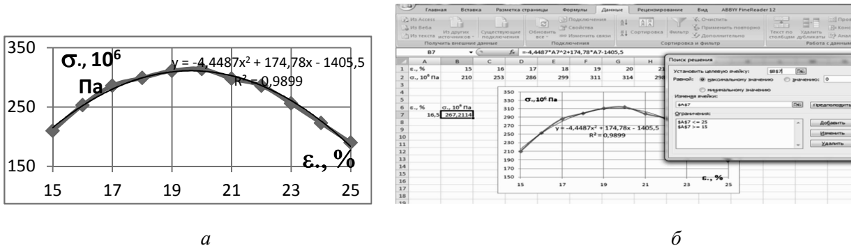
Рис. 3. Расчет предельных деформаций и предела прочности материала с помощью функции-оптимизатора (а – вид тренда для экспериментальной кривой; б – этап решения)
