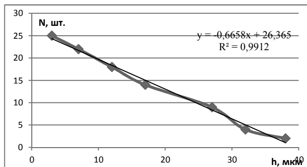
Рис. 5. Зависимость количества выявленных питтингов от глубины визуализации
