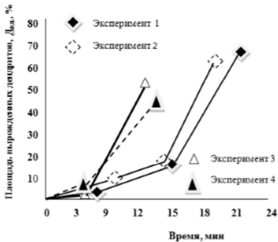
Рис. 1. Влияние УЗО на степень вырождения дендритной структуры твердого раствора сплава АК7
