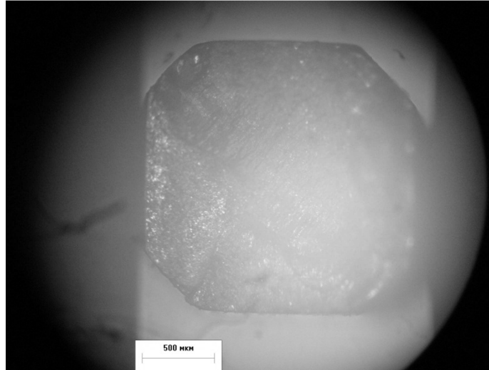
Рис. 3. Поперечное сечение образца деформированного никелида титана после разрушения под действием УЗО
