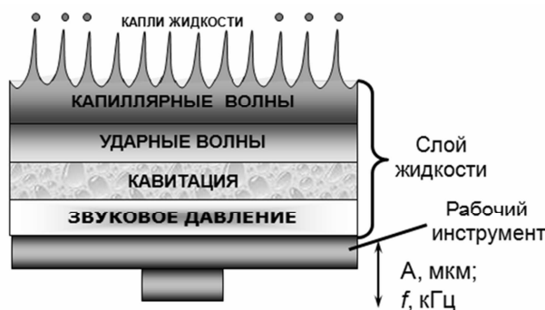
Рис. 1. Схематичное изображение кавитационно-волнового механизма образования капель в слое распыляемой жидкости
