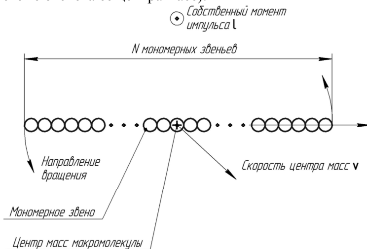
Рис. 1. Линейная модель макромолекулы.
