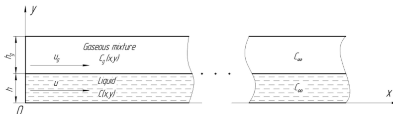
Рис. 1. Модельная двухслойная система «жидкость-газ» для теоретического анализа кинетики абсорбции
