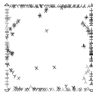
Рис. 3. Расположение дислокаций в расчетной ячейке после ультразвукового воздействия в течение 5000 периодов колебаний при значениях параметров K=0.5 и Q=0.5 .
