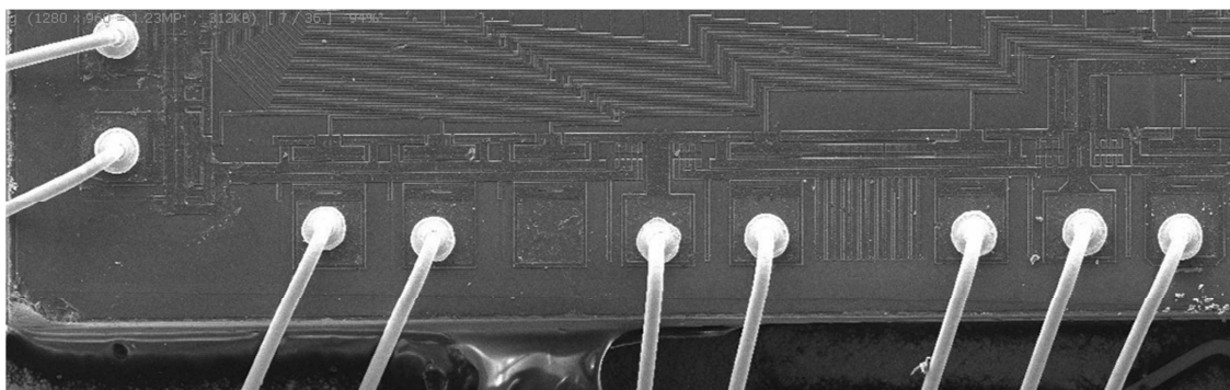
Рис. 1. Проволочные соединения золотой проволокой методом «шарик-клин»
