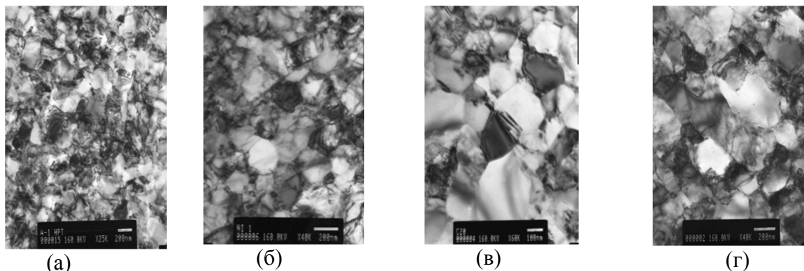
Рис. 2. Микроструктура образцов после КГД (а), после УЗО с медными подкладками без смазки (б) и со смазкой (в) и с баббитовыми подкладками (г).
