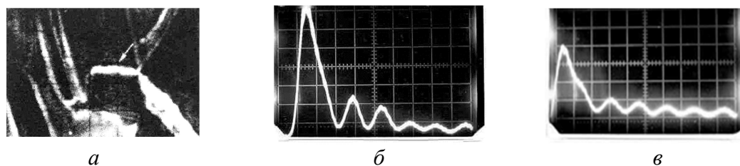
Рис. 5. Обнаружение дефектов металлических материалов после деформации; а - акустическое изображение трещины в стали аустенитного класса ( Z = -40 мкм, масштаб 20 мкм/дел.); б - V(Z) -кривые для одного из сортов стали (изменяется форма в районе микротрещины; ст. 30ХГСМЛ, v_R = 3,18 \cdot 10^3 м/с, \Delta Z_N = 14,68 мкм, (\Delta V/V\%)_{\text{max}} = 37\% , масштаб по вертикали 1 дел.= 0,25 В, по горизонтали – 1 дел.=12,2 мкм).
