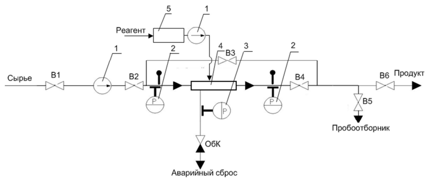
Рис. 2. Аппаратурно-технологическая схема гидродинамической проточной установки: 1 – насос, 2- манометр, 3 - моновакуумметр, 4 – гидродинамический кавитационный модуль, 5 – блок предварительной УЗ - активации реагента.
