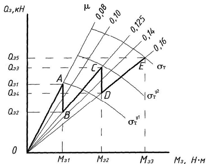
Рис. 2. Изменение силы затяжки крепёжной детали в зависимости от прикладываемого крутящего момента при ультразвуковой сборке: \sigma_T и \sigma_B - предел текучести и прочности при обычной сборке, \sigma_T^y и \sigma_B^y - предел текучести и прочности при ультразвуковой сборке
