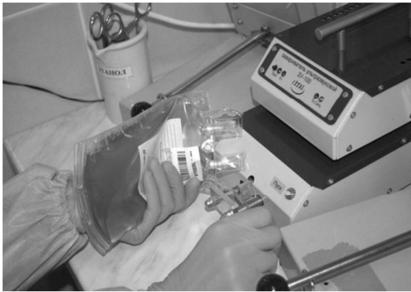
Рис. 2. Аппарат для ультразвуковой сварки магистралей систем переливания крови
