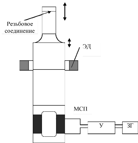
Рис. 1. Блок-схема установки для экспериментального исследования влияния ультразвуковых колебаний на усилие разборки резьбовых соединений
