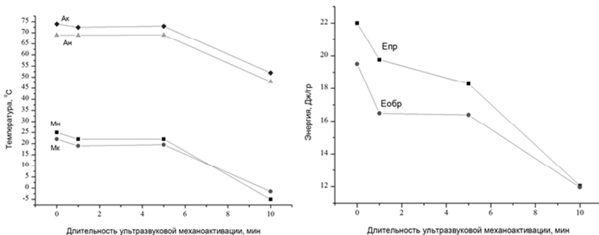
Рисунок 3- Зависимости температур мартенситных превращений (а) и энергий (б), выделившихся при прямом и обратном превращениях
