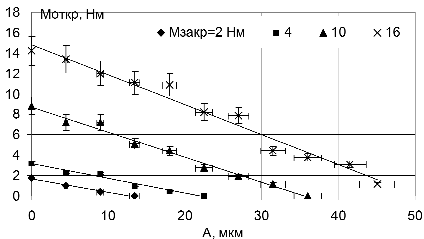
Рис. 3. Зависимости момента откручивания от амплитуды продольных колебаний при различных моментах закручивания
