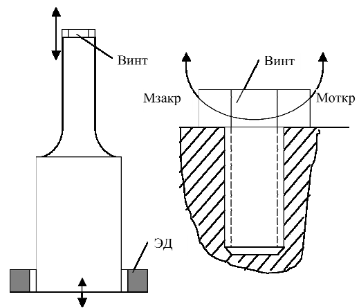
Рис. 2. Выходная полуволна колебательной системы и исследуемое резьбовое соединение
