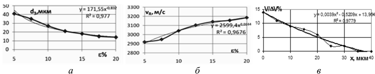
Рис. 4. Корреляционная зависимость (а) размера зерна от степени деформации (ст. 20ХГСА); б) Зависимость скорости ПАВ от степени деформации (ст. 20ХГСА); в) изменение коэффициента затухания АВ в меди с трещиной после деформационного воздействия
