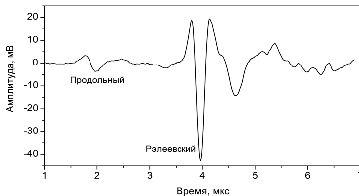
Рис. 3. Пример опико-акустического сигнала, зарегистрированного в образце никеля.
