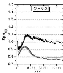
Рис. 2. Зависимость изменения относительного значения среднеквадратичного следа напряжений, рассчитанная для одной и той же системы, от времени ультразвукового воздействия
