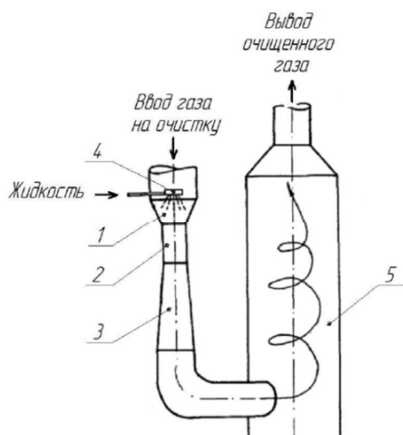
1 – конфузор; 2 – горловина; 3 – диффузор; 4 – форсунка; 5 – циклон-каплеуловитель Рис. 4. Схема скруббера Вентури
