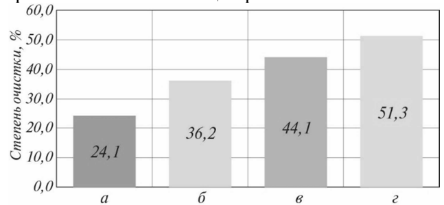
Рис. 3. Повышение эффективности применения Аква-Аурата 30 и Праестола 857 при их совместном использовании и предварительной УЗ активации (УЗА): а – Аква-Аурат А30; б – Аква-Аурат А30 и Праестол 857; в – то же, Праестол подвергался УЗА в течение 10 с; г – то же, Аква-Аурат А30 подвергался УЗА в течение 30 с, а Праестол в течение 10 с
