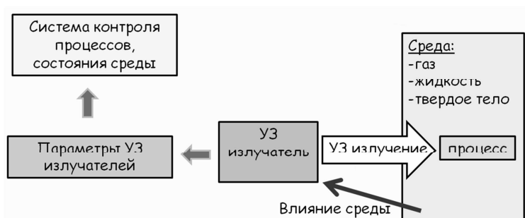
Рисунок 2 – Схема косвенного контроля технологических процессов и явлений, протекающих в УЗ полях
