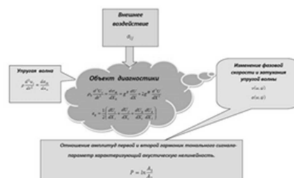
Рис. 4. Методология оценки поврежденности по акустической нелинейности.
