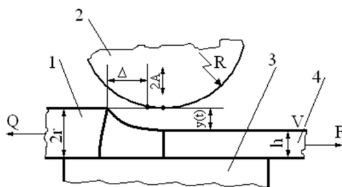
Рис. 1. Схема деформирующего узла
