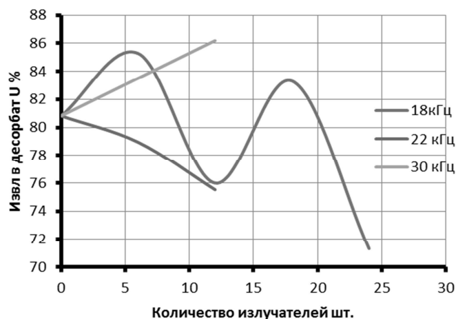
Рис 3 - Изменение извлечения урана в десорбат в зависимости от количества работающих излучателей
