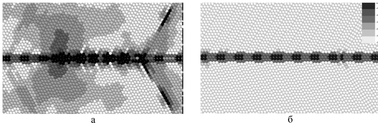
Рис. 2. Карты атомных напряжений в бикристалле, содержащем границу наклона \Sigma = 11 [112] с дисклинационным диполем, до (а) и после (б) воздействия ультразвука
