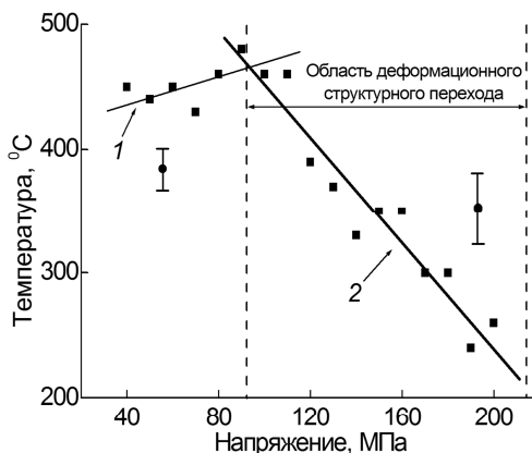
Рис. 2. Зависимость критической температуры деформационного структурного перехода от механического напряжения в циклах.
