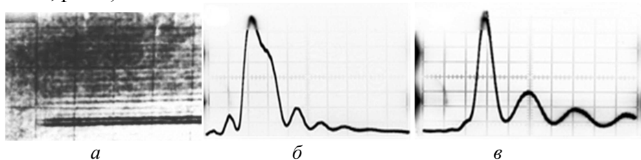
Рис. 1. Анализ дефектных структур АМД-методами a - акустическое изображение микротрещины в полупроводнике ( \text{Si}\langle 111 \rangle , масштаб 20 мкм/дел., f = 402 МГц, Z = -16 мкм); б, в - V(Z) -кривые для полупроводниковых материалов (германий ( б ) и кремния( в ), (масштаб по вертикали 0,4 В, по горизонтали, соответственно, 1 дел.=11 мкм и 16 мкм).
