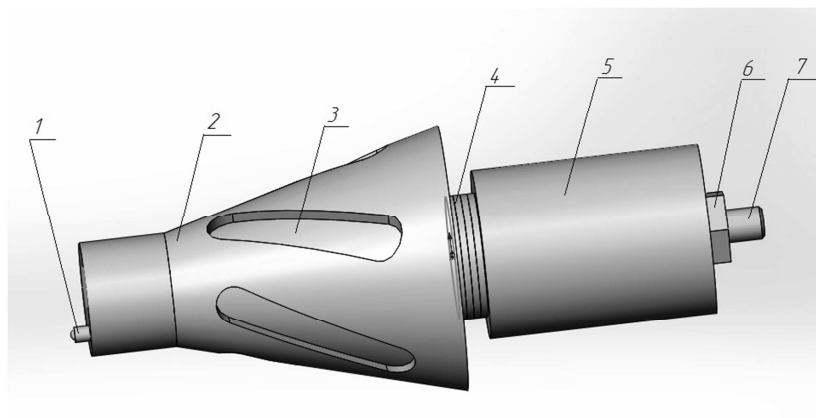
Рис. 1. Ультразвуковое устройство для формирования микрорельефа поверхностей
