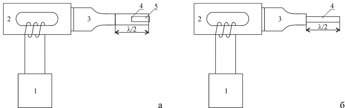
Рис. 1. Принципиальные схемы ультразвуковой обработки дисковых (а) и цилиндрических полуволновых (б) образцов: 1 – ультразвуковой генератор; 2 – преобразователь; 3 – концентратор; 4 – образец, 5 – прижимной цилиндр
