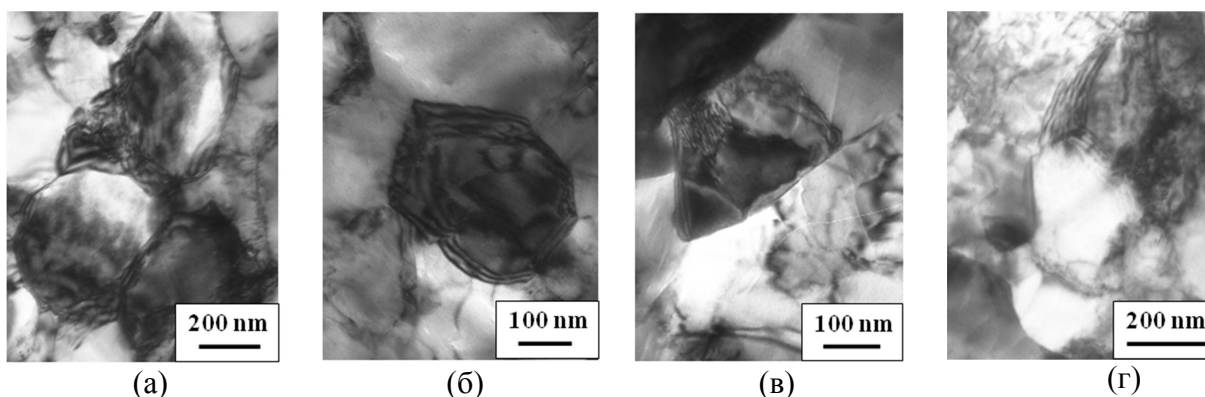
Рис. 2. Микроструктура образцов никеля, подвергнутых КГД (а) и УЗО с амплитудами 20 (б), 40 (в) и 60 МПа (г)
