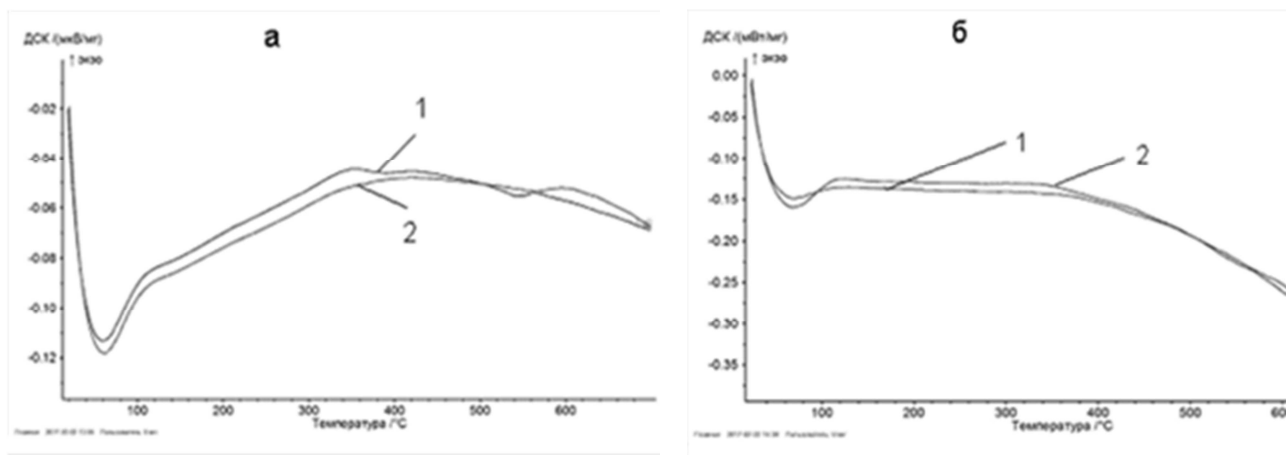
Рис. 4. Кривые ДСК образцов сплава Ti-50,7ат.%Ni после прокатки с током до \epsilon=1,2 (а) и последующей УЗО (б); кривые 1 – первый цикл нагрева, кривые 2 – повторный нагрев
