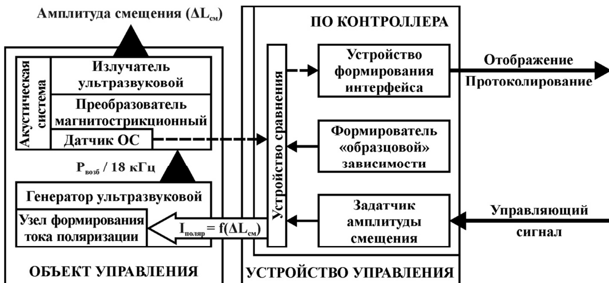
Рис. 1. Структурная схема следящей системы
