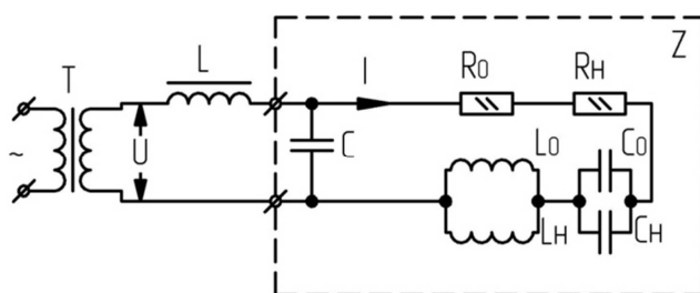
Рисунок 1 – Эквивалентная электрическая схема замещения УЗКС с пьезоэлектрическим преобразователем
