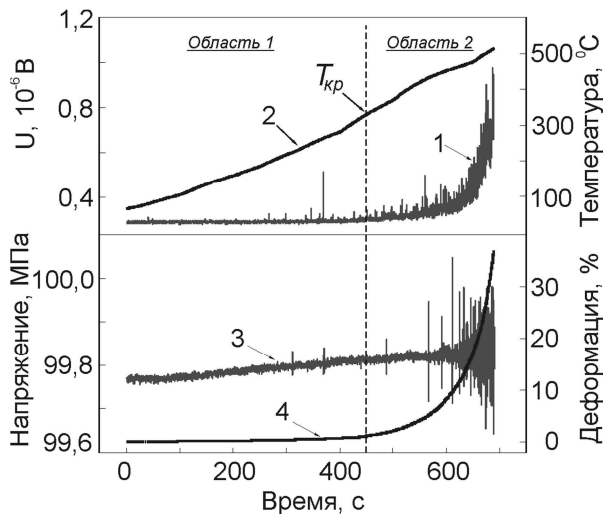
Рис. 1. Акустическая эмиссия (1), температура (2), механическое напряжение (3) и накопление деформации (4) при нагреве образца АМг5 в условиях действия постоянной нагрузки 100 МПа.
