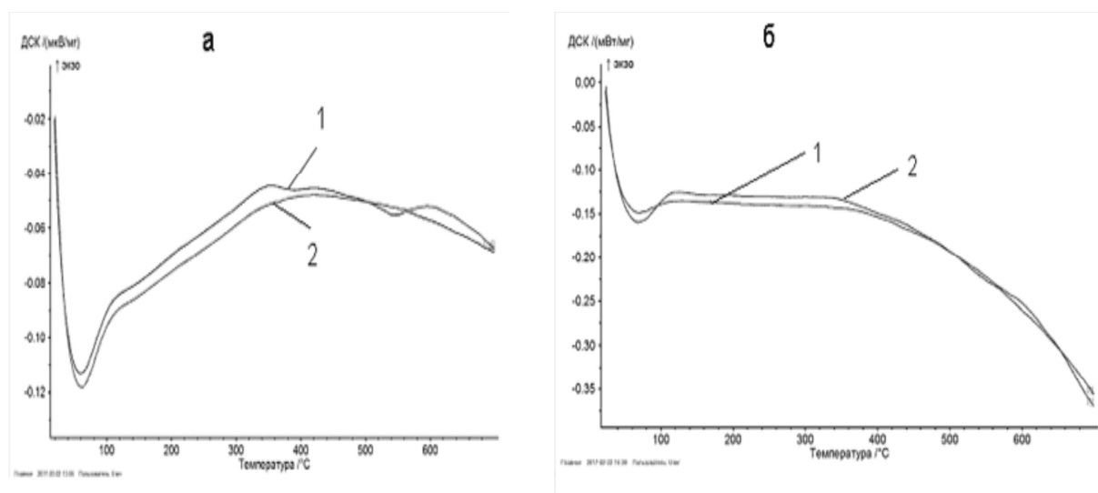
Рис. 2. Кривые ДСК образцов никелида титана после прокатки (а) и последующей ультразвуковой обработки (б); кривые 1 - первый цикл нагрева, кривые 2 - повторный нагрев
