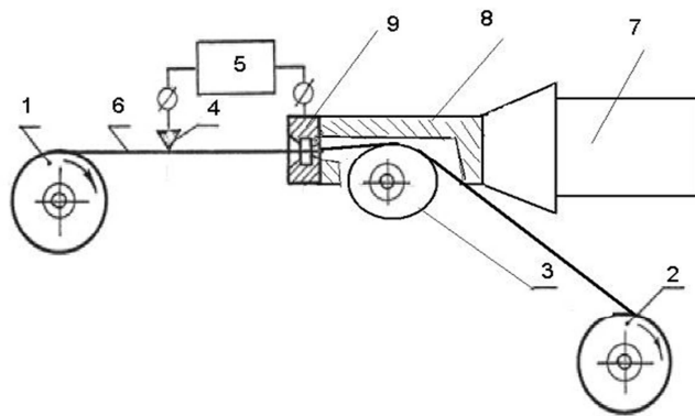
Рис. 1. Устройство волочения и воздействия на проволоку ультразвуковых колебаний: 1- отдающий барабан, 2 – тянущее устройство, 3 – направляющий ролик, 4 – контактное устройство, 5 – генератор электрических импульсов, 6 – обрабатываемая проволока, 7 – ультразвуковой преобразователь, 8 – волновод, 9 – фильера
