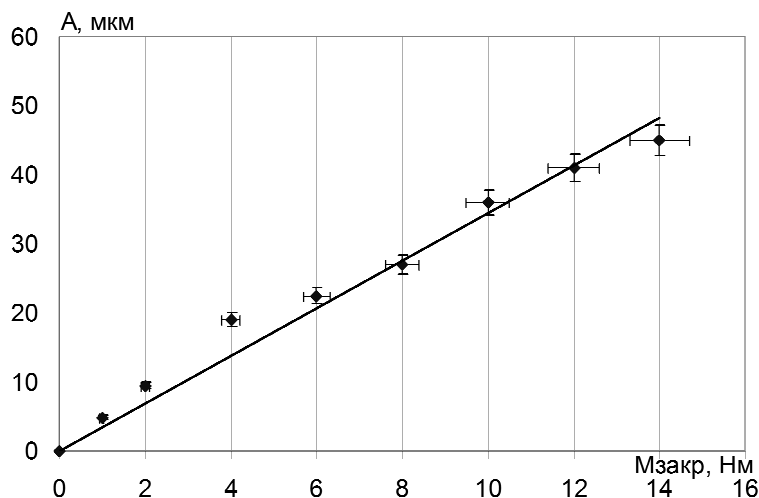
Рис. 4. Зависимость амплитуды ультразвуковых колебаний, при которой происходит самооткручивание резьбового соединения, от усилия его закручивания
