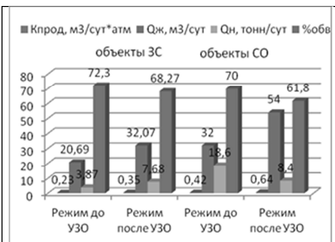
Рис. 1. Влияние УЗО на параметры работы скважины с учетом отработанного времени
