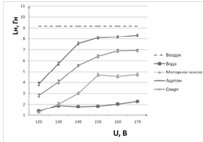
Рисунок 4 – Зависимость индуктивной части импеданса механической ветви УЗКС от возбуждающего напряжения
