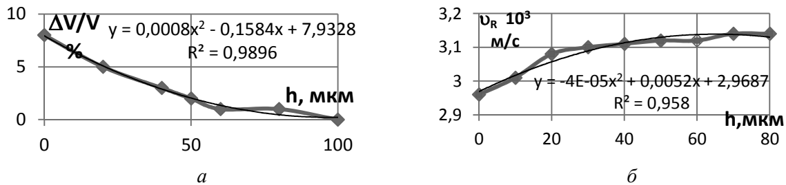
Рис. 6. Характеризация дефектных структур в стали с помощью АМД-методов; a - изменение уровня затухания АВ в образце с глубиной зондирования; б - изменение скорости ПАВ в образце с увеличением толщины снятого слоя.
