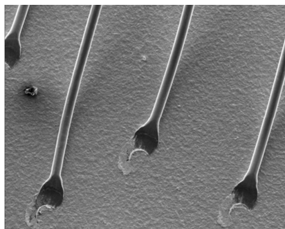
Рис. 4. Вид соединений шариком встык при использовании ультразвуковой частоты 110 кГц
