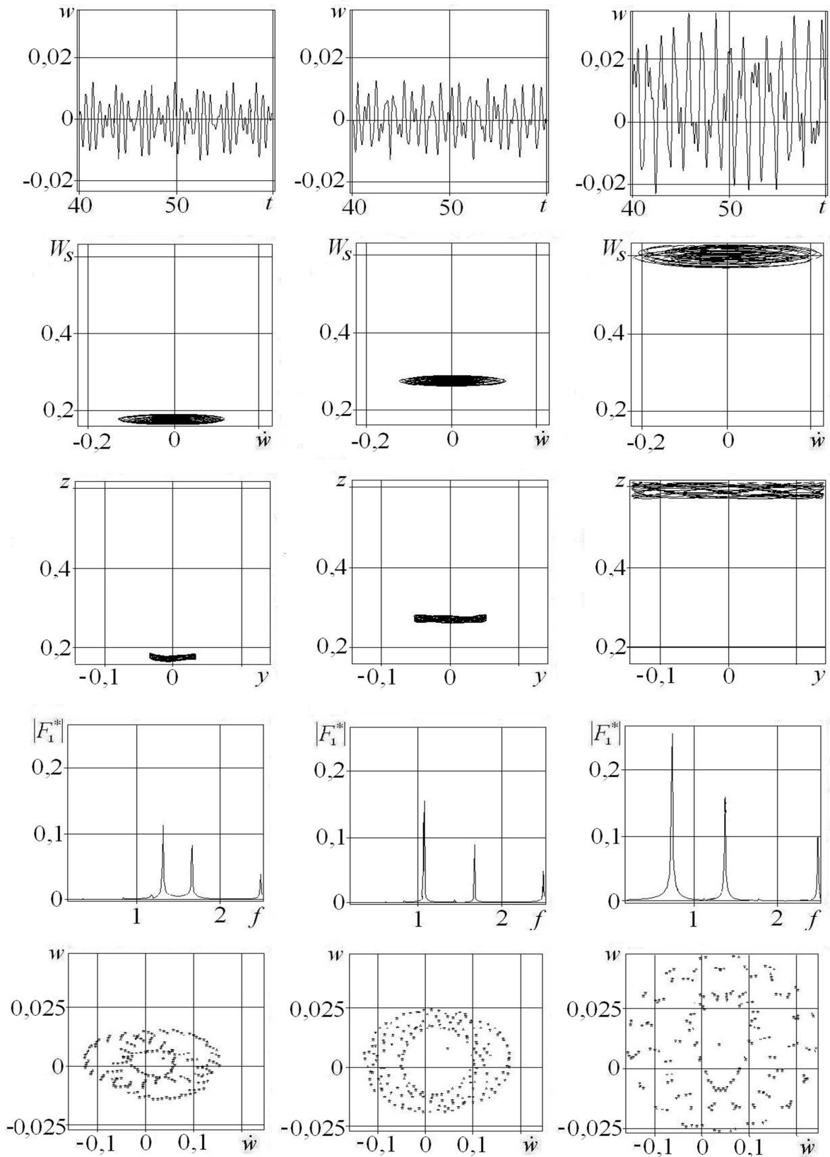
Рис. 1. Зависимости динамической составляющей прогиба w , м, от времени t , с, фазовые траектории, W_s , м, \dot{w} , м/с, проекция траектории средней точки пролета с координатами x , y , z , м, на вертикальную плоскость y z , спектры частот, |F_1^*| , м·с, и отображения Пуанкаре изгибных колебаний трубы в воздушной среде при частоте f = 2.5 Гц, амплитуде p_a = 0.15 МПа, начальной фазе \varphi_0 = 0 рад и разных значениях p_0 переменного внутреннего давления
