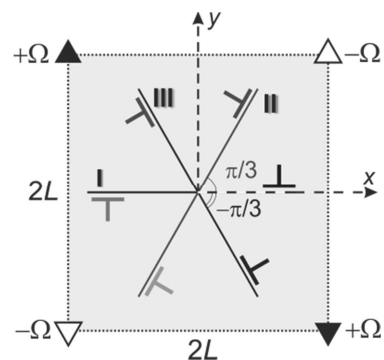
Рис. 1. Схематическое изображение модельного квадратного зерна с тремя плоскостями скольжения.
