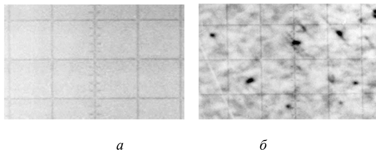
Рис. 4. Оптическое (а) 210^x и акустическое (б) изображения приповерхностного слоя стали (08X21H6M2T), подвергнутой коррозионным испытаниям (б - питтинг, масштаб 35 мкм/дел., f = 402 МГц, Z = -2 мкм)
