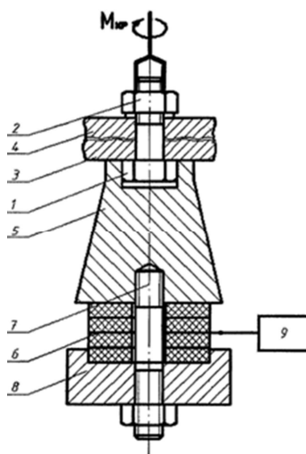
Рис. 1. Структурная схема устройства для реализации ультразвуковой сборки резьбовых соединений
