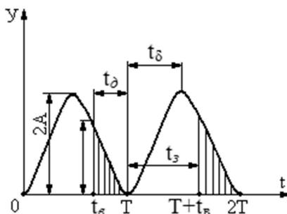
Рис. 2. Кинематика процессаковки:
