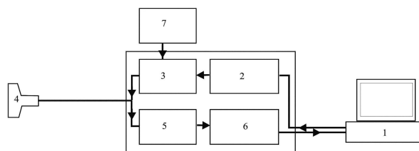
Рис.1 б. Блок-схема исследовательской акустической системы Verasonics
