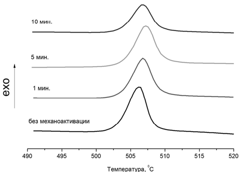
Рисунок 1 - Калориметрические кривые, полученные при нагреве аморфного сплава
