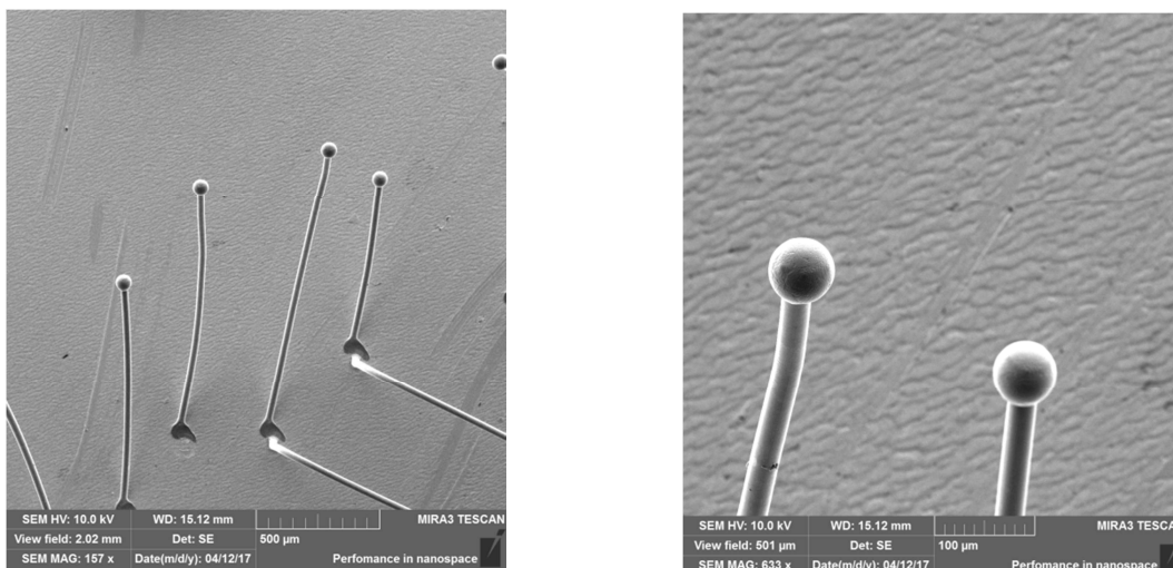
Рис. 2. Оплавленные шарики на кончике медной проволоки
