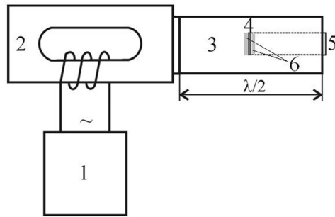
Рис. 1. Схема ультразвуковой обработки никеля, подвергнутого кручению под высоким давлением. 1-генератор ультразвуковых колебаний, 2-преобразователь, 3-концентратор, 4-образец, 5-прижимной цилиндр, 6-подкладки.
