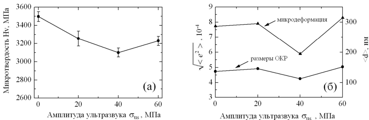
Рис. 1. Зависимость микротвердости (а), среднеквадратической микродеформации и размеров ОКР (б) образцов никеля, подвергнутых КГД, от амплитуды УЗО
