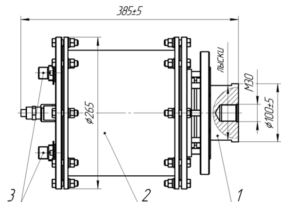
Рис. 5. Эскиз УЗ колебательной системы для возбуждения колебаний физических объектов: 1 – рабочий инструмент, 2 – пьезоэлектрический преобразователь в корпусе, 3 – патрубki для жидкостного охлаждения
