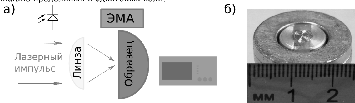
Рис. 1. Схема эксперимента (а), ЭМА-преобразователь (б).
