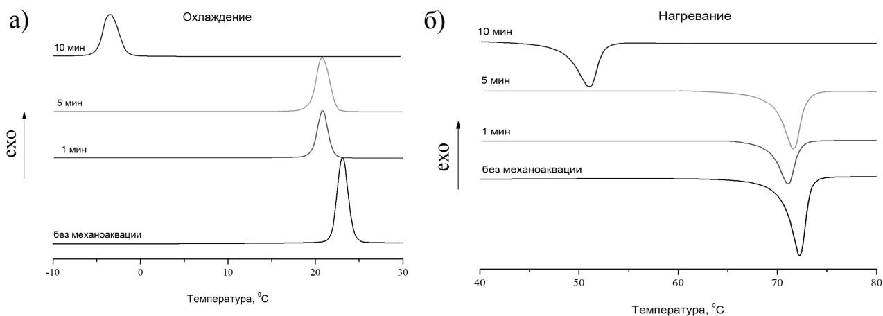
Рисунок 2- Калориметрические кривые мартенситных превращений аморфного сплава при охлаждении (а) и нагревании (б)
