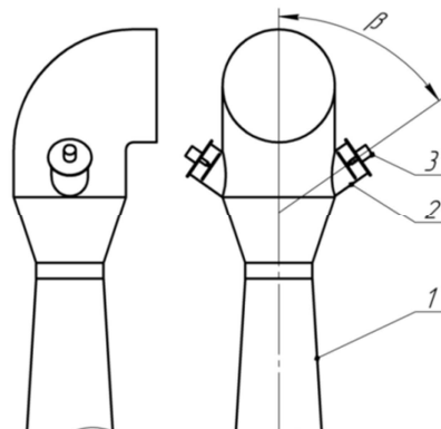
1 – труба Вентури; 2 – отвод для установки УЗ-излучателя; 3 – УЗ-дисконный излучатель; Рис. 5. Схема установки 2-х УЗ-излучателей в трубу Вентури
