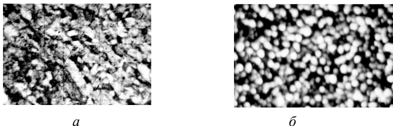
Рис. 1. Акустические изображения; а - структуры стали, позволяющее рассчитать прочностные свойства стали по размеру зерна (масштаб: 20 мкм/дел., Z = - 17 мкм), б - строение пьезокерамики ЦТС-19 на глубине ~32 мкм (частота 404 МГц, размер по горизонтали 250 мкм)
