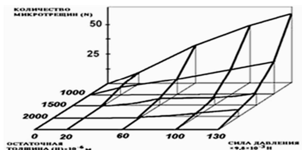
Рис. 3. Корреляция числа дефектов в стекле и параметров обработки (по результатам АМД-методов). Экспериментальная зависимость для стекла ТПС числа выявленных микронеоднородностей N от силы давления F на образец и глубины визуализации H
