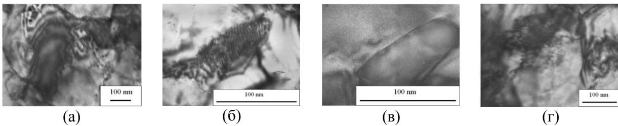
Рис. 2. ПЭМ-изображения дефектной структуры УМЗ никеля после КГД (а) и УЗО с амплитудами 15 (б), 60 (в) и 90 МПа (г)
