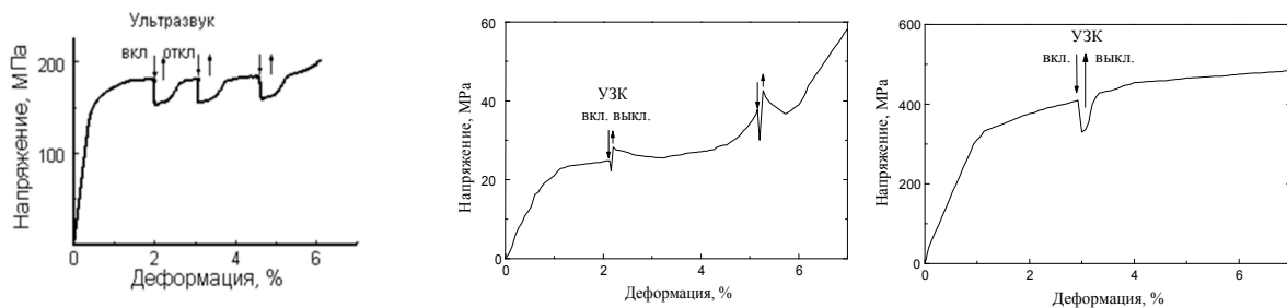
Рис. 5. Диаграммы растяжения Ti-50,8 ат.% Ni проволоки, включающие импульсное воздействие ультразвука ( A_n=17^\circ\text{C} , A_k=22^\circ\text{C} , M_n=33^\circ\text{C} , M_k=55^\circ\text{C} , M_k=10^\circ\text{C} ), амплитуда УЗК - 5 мкм
