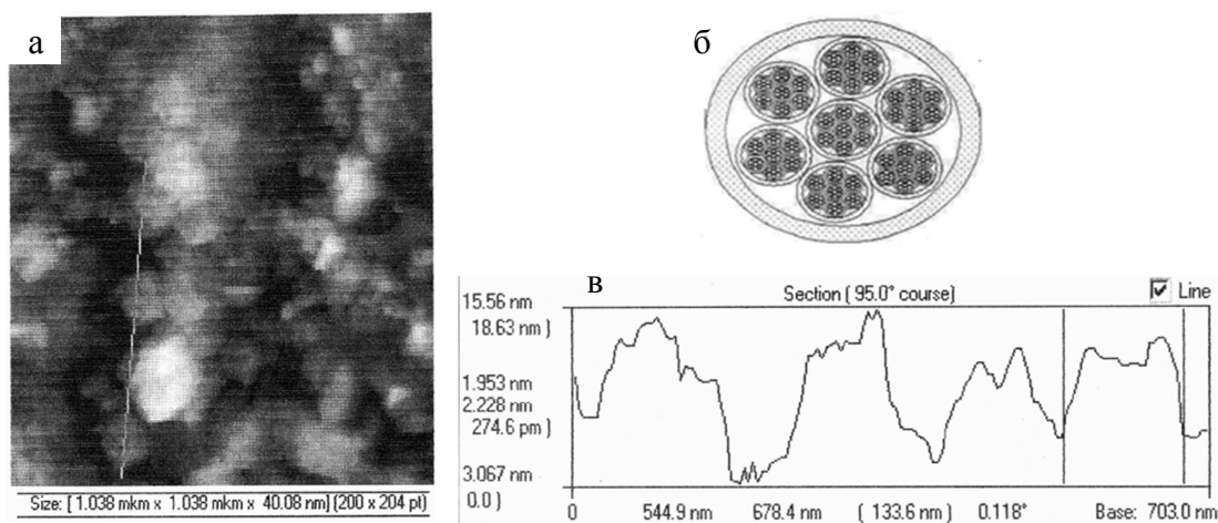
Рис. 2. Электронномикроскопическое исследование нановолокнистого Cu-NbTi композита с участком трассирования электронного луча (а); геометрия торцевой поверхности (б); профилограмма торцевой поверхности разрыва (в).
