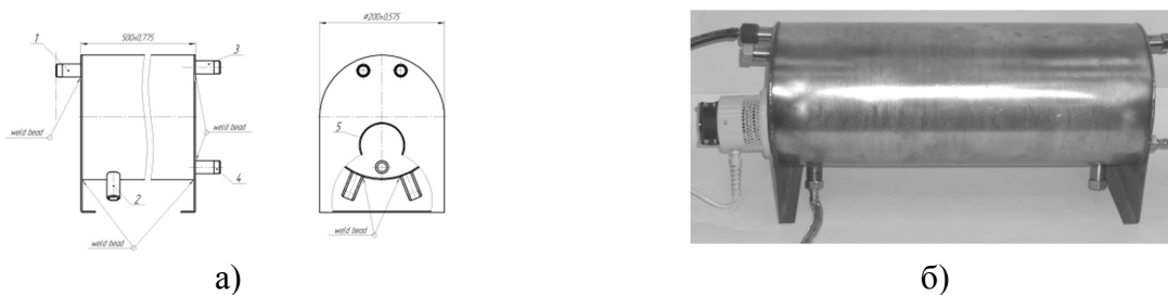
Рис. 2. Эскиз (а) и фото (б) технологического объёма для протекания абсорбции с установленным ультразвуковым излучателем
