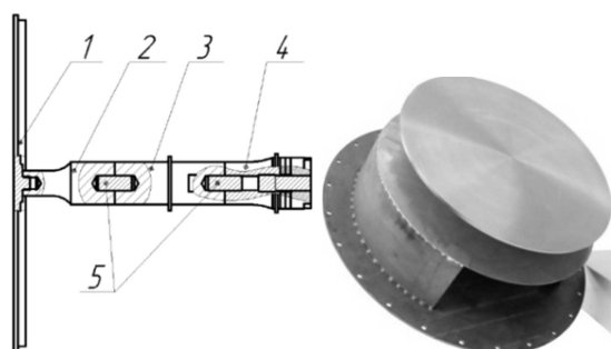
1 – дисковый излучатель; 2 – концентратор; 3 – волновод; 4 – пьезоэлектрический преобразователь; 5 – шпильки
