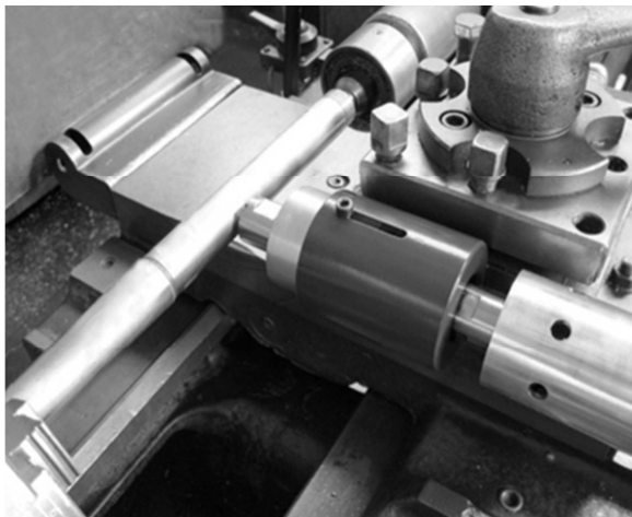
Рис. 4. Устройство для ультразвуковой поверхностной обработки
